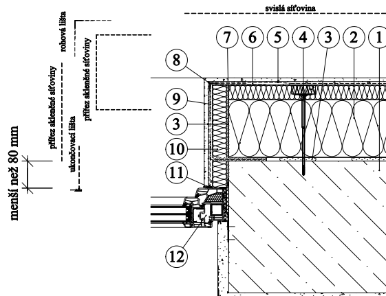
- detail pro ostění
