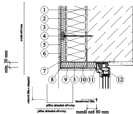
- detail pro nadpraží
