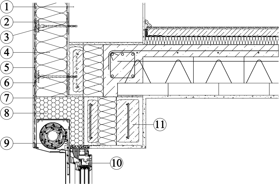
Fasádní tepelně izolační desky z minerální vlny KNAUF INSULATION - SMARTwall S C1, SMARTwall S C2, FKD S Thermal - šroubovací hmoždinka SMARTfix S - v zateplovacím systému ETICS - s oboustranným silikátovým nástřikem - nadpraží okna/dveří s venkovní roletou - VARIO - překlad 7
