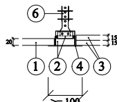
řez B-B Detail C - příčný řez nosný profil pro rastrový páskový strop
