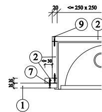
řez F-F Detail G - kruhové svítidlo
