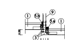
Detail L - mezilehlé zavěšení s výškovým přesazením stropu
