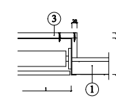
Detail O - vestavné svítidlo - podélný řez
