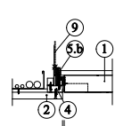
Detail K - výškové přesazení
