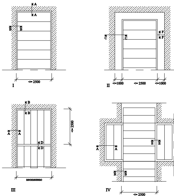
Detail A - stropní pohledy, varianty
