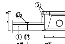
Detail N - vestavné svítidlo - příčný řez
