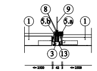
Detail I - mezilehlé zavěšení
