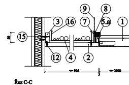
Detail C - sklopné kovové stropní prvky, připojení ke stropnímu výslu
