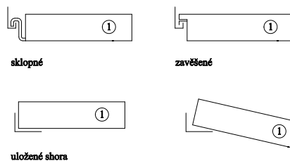
Detail B - sklopné, zavěšené a shora uložené kovové stropní prvky
