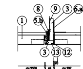
Detail J - zavěšení pro zaústění chůby
