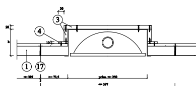
Detail P - kruhové svítidlo, příčný řez
