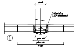
Detail Q - příčný řez VZT ventilem
