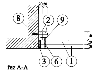
řez A-A Detail B - připojení ke stěně
