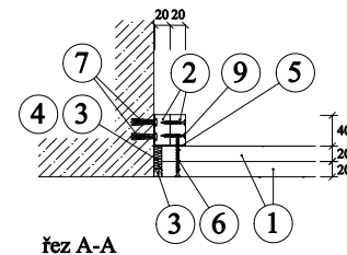
řez A-A Detail B - připojení ke stěně
