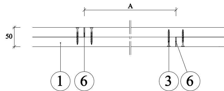
Detail B - umístění spoje
