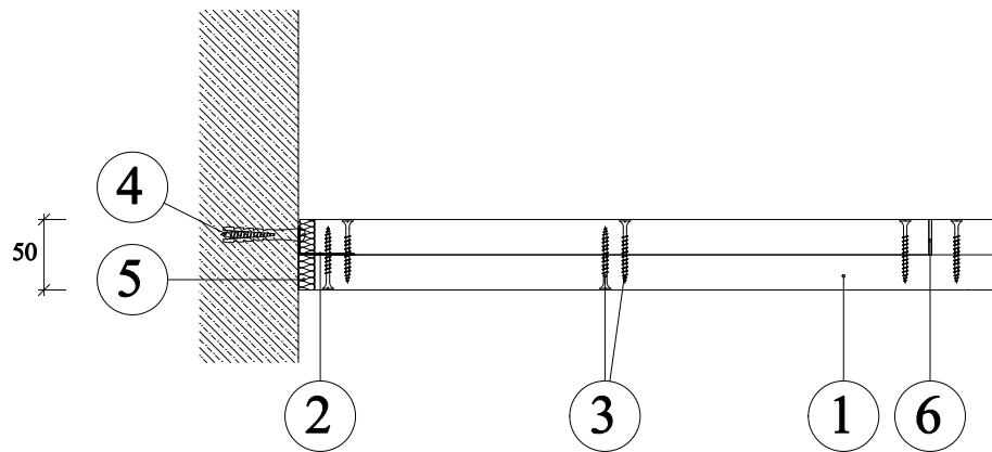
Detail A - připojení ke stěně
