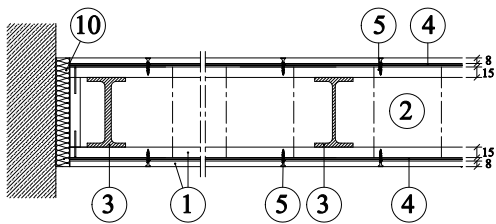
Detail A - horizontální řez - možné uspořádání ocelových plechů
