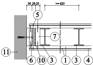
Řez A-A:
