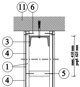
Řez C-C - připojení k podlaze a ke stropu:
