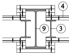
Řez B-B:
