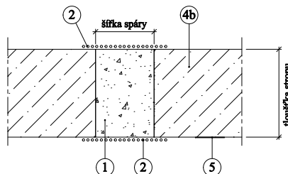
Detail F - vodorovná spára ve vodorovné konstrukci
