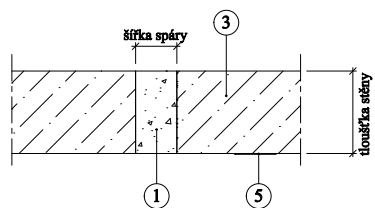
Detail A - pohled shora - svislá spára ve svislé konstrukci
