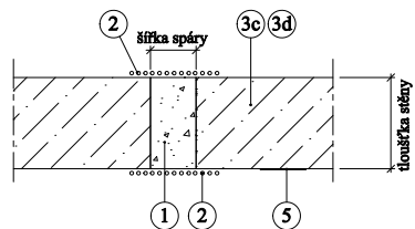
Detail D - pohled shora - svislá spára ve svislé konstrukci
