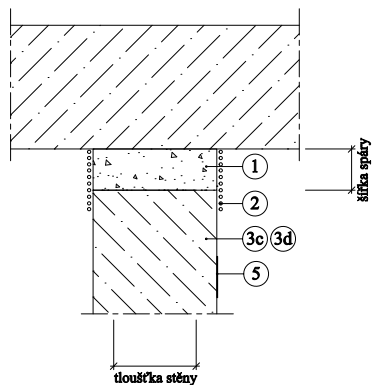
Detail E - vodorovná spára ve svislé konstrukci
