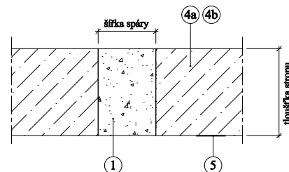
Detail C – vodorovná spára ve vodorovné konstrukci
