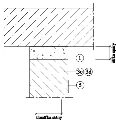
Detail B – vodorovná spára ve svislé konstrukci
