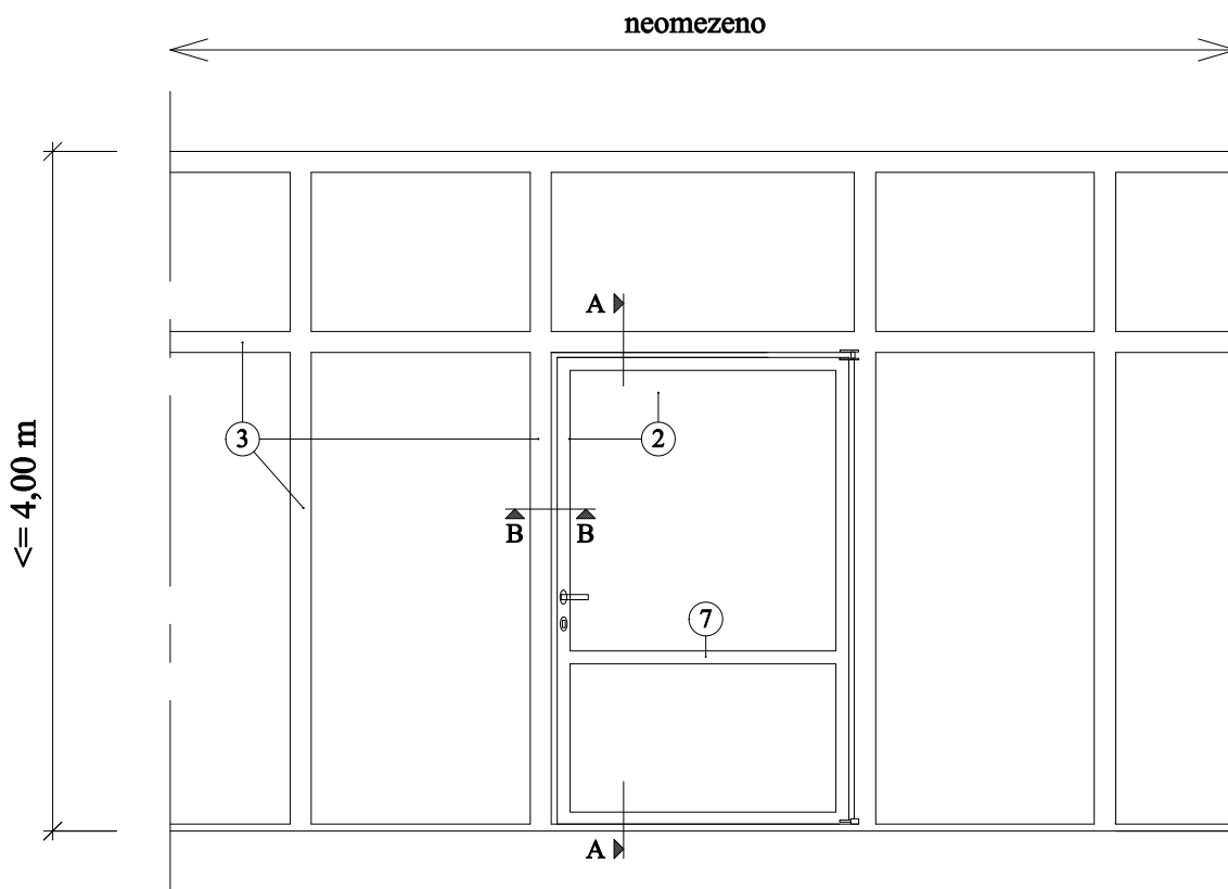
Detail A - pohled
