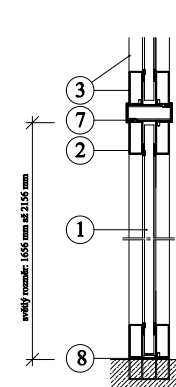
Detail B - svislý řez A-A
