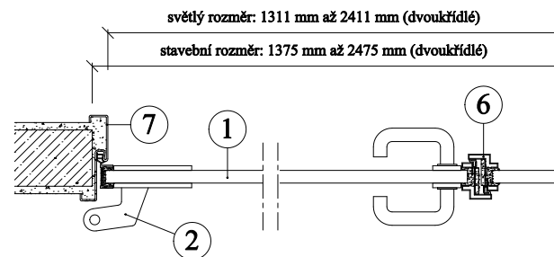
Detail C - vodorovný řez A-A
