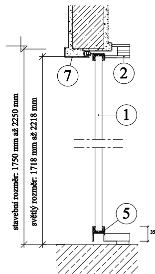
Detail C - svislý řez B-B
