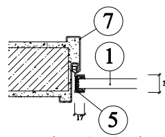
Detail B - rohová zárubeň s dorazem dveří
