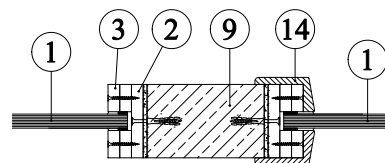
Detail C - masivní sloupek
