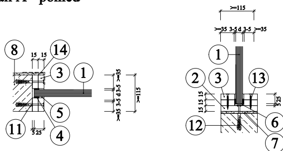
Detail B - vestavba do masivní stěny
